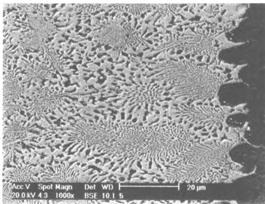
FIGURA 2.- Detalle de la sección transversal de la pieza nº 5 (1000 x), bajo el microscopio de barrido. La zona corresponde a la cobertura de plata, donde podemos observar las estructuras eutécticas formadas a partir de la introducción del flan de cobre en un baño de plata fundida.
